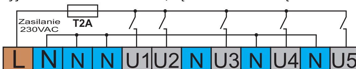
Wyjścia U1...U5: 230VAC, łączna moc obciążenia 400W
