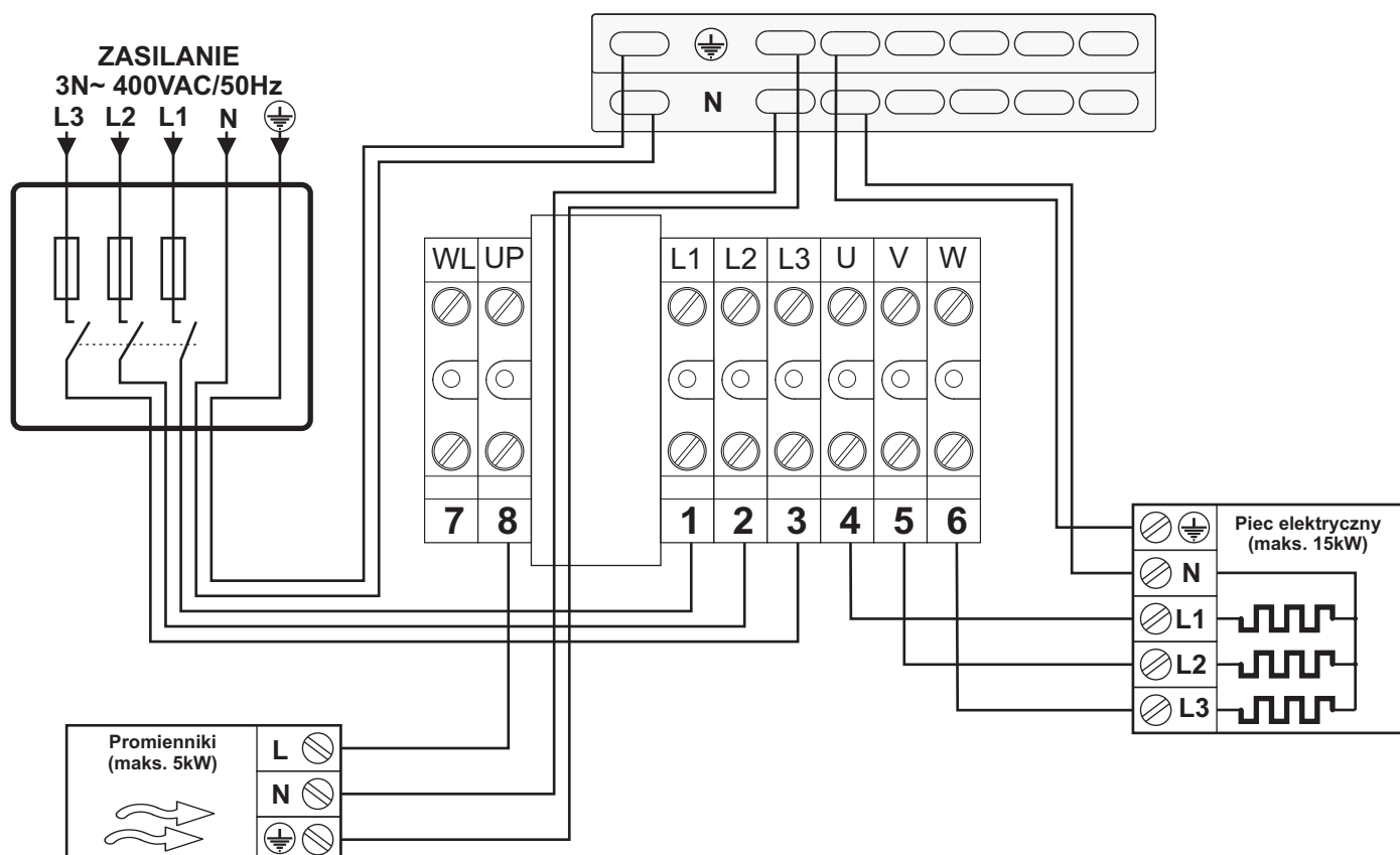
S3. Schemat podłączenia pieca elektrycznego i promienników. Funkcje sterujące F30, F31, F32, F33.
