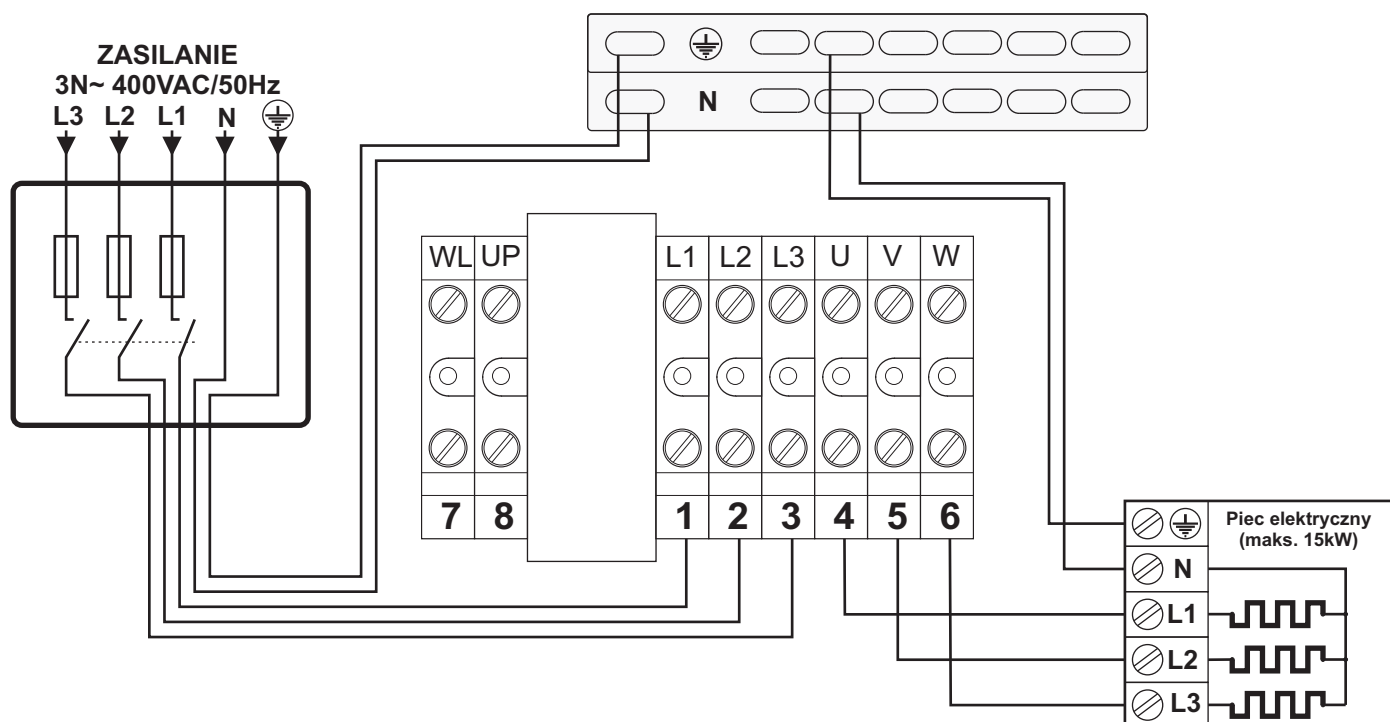
S2. Schemat podłączenia pieca elektrycznego. Funkcje sterujące F10, F11, F12, F13.
