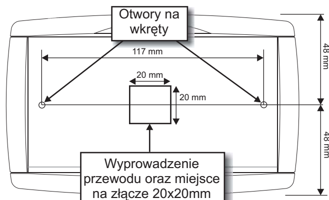
Rozstaw otworów montażowych panelu na ścianie
