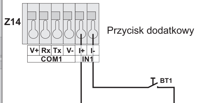
Schemat podłączenia wejścia DIN
