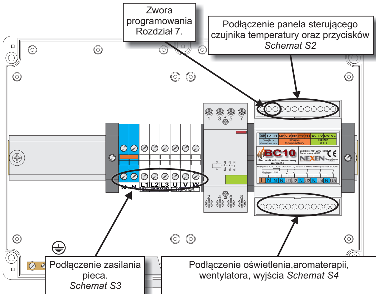
S1. Widok modułu sterownika po zdjęciu pokrywy górnej.
