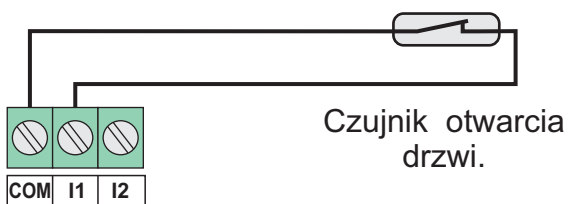
Schemat podłączenia czujnika otwarcia drzwi do wejścia IN1.
