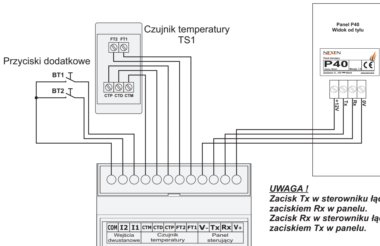
S2. Schemat podłączenia czujnika temperatury TS1, panelu sterującego i przycisków.
