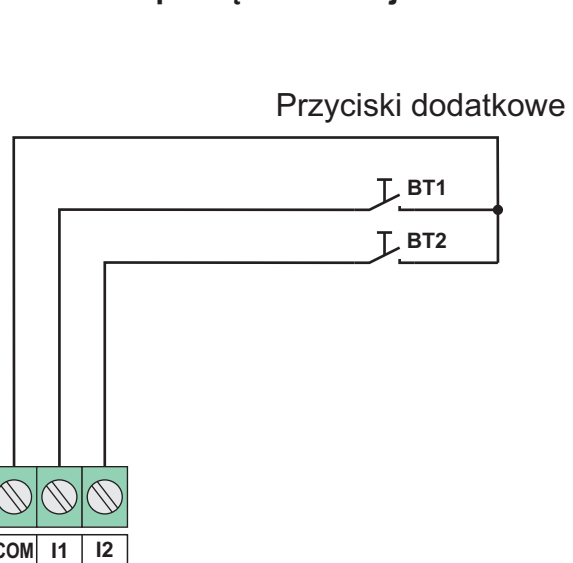
Schemat podłączenia wejść DIN
